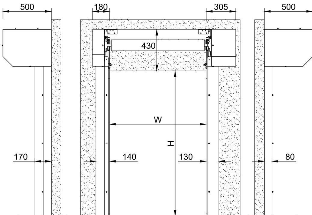
Установочные размеры ворот DZ/F-DZ
