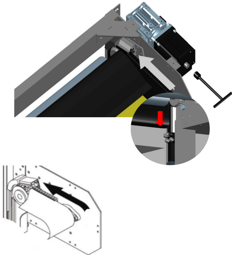
Рис 5-5: Заправка полотна ворот
