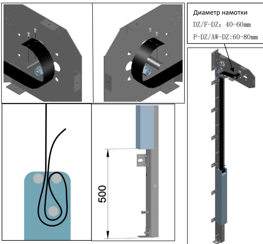
Рис 5-6: Установка противовеса
