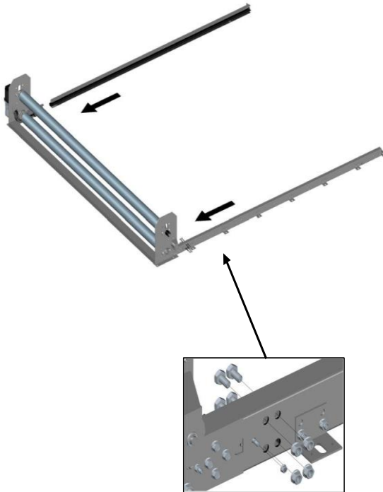
Рис5-1: сборка ворот на полу
