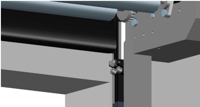
Рис 5-9: настройка верхних зазоров полотна
