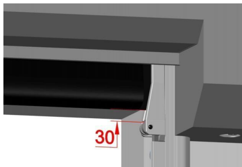
Рис.5-8: Настройка верхнего положения полотна ворот
