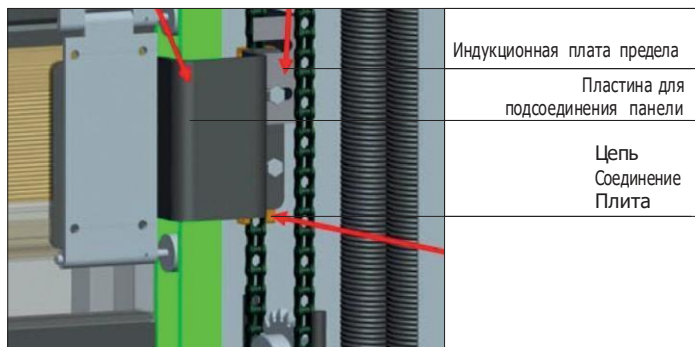
2. Место установки электромагнитного концевого выключателя.
