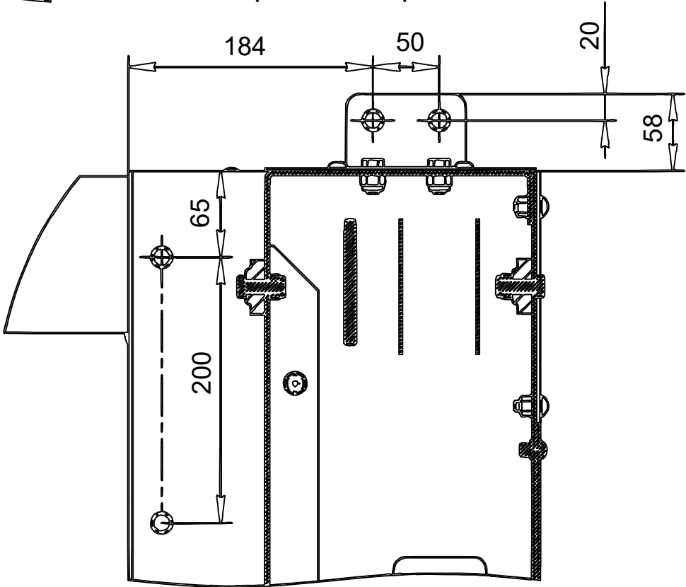
Крепление верхнего узла спирального кронштейна
